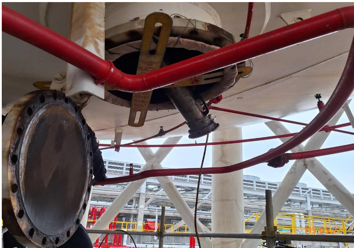
5. 球槽底部開完人孔情形
