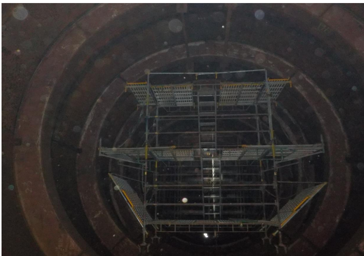
8. 槽內搭架作業情形(5)
