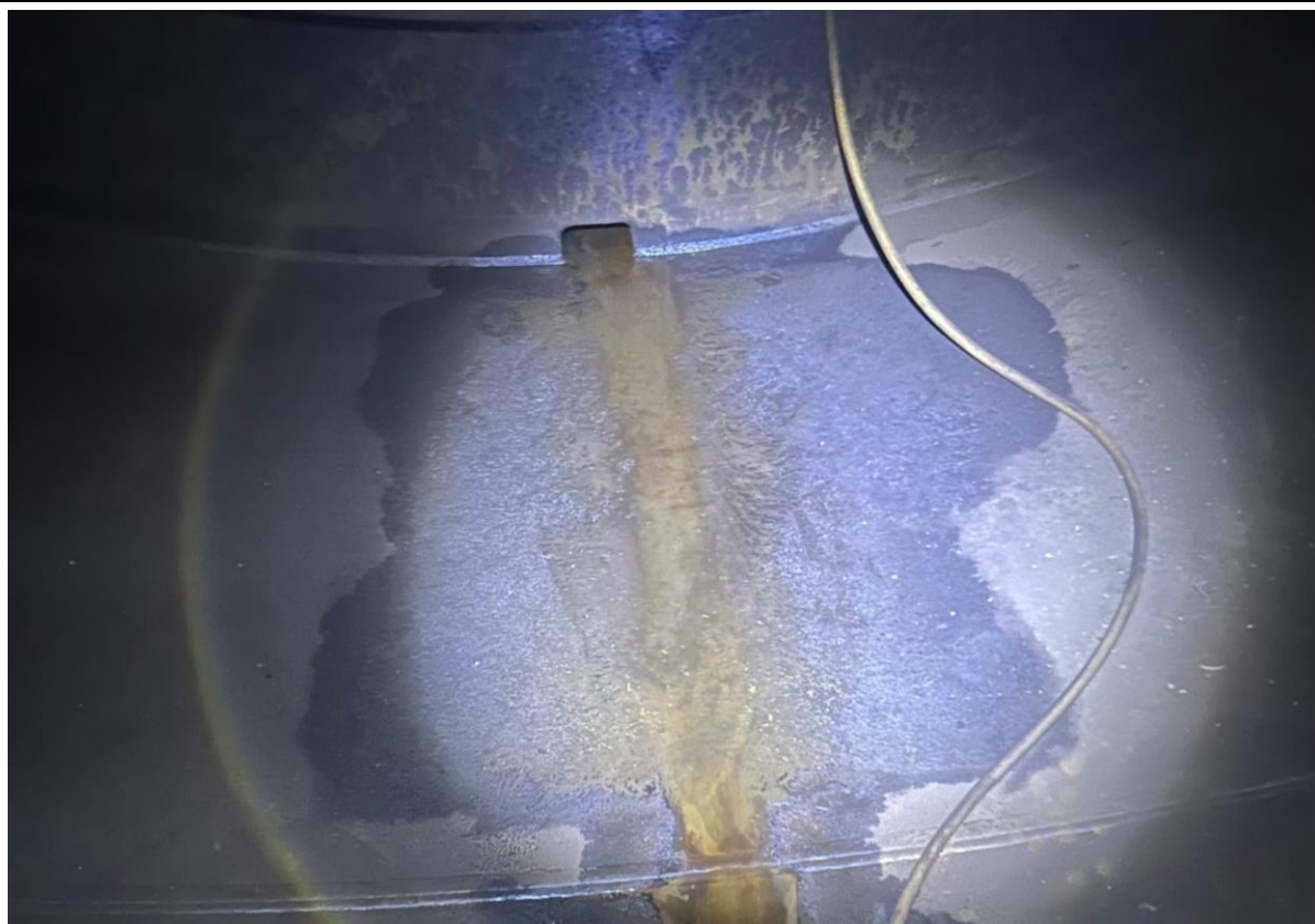
11. 槽內焊道研磨(3)
