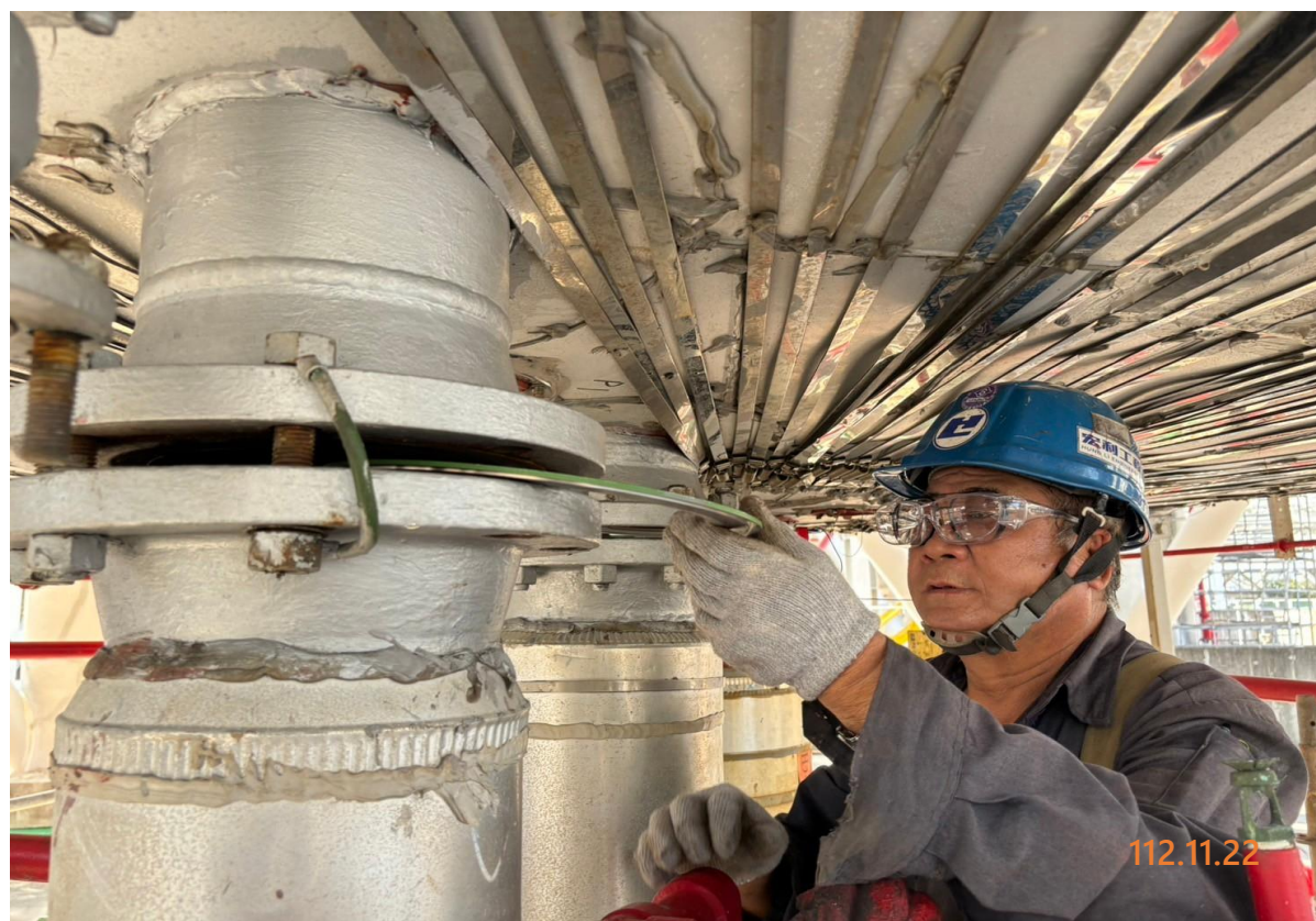
15. 管線抽盲作業(1)
