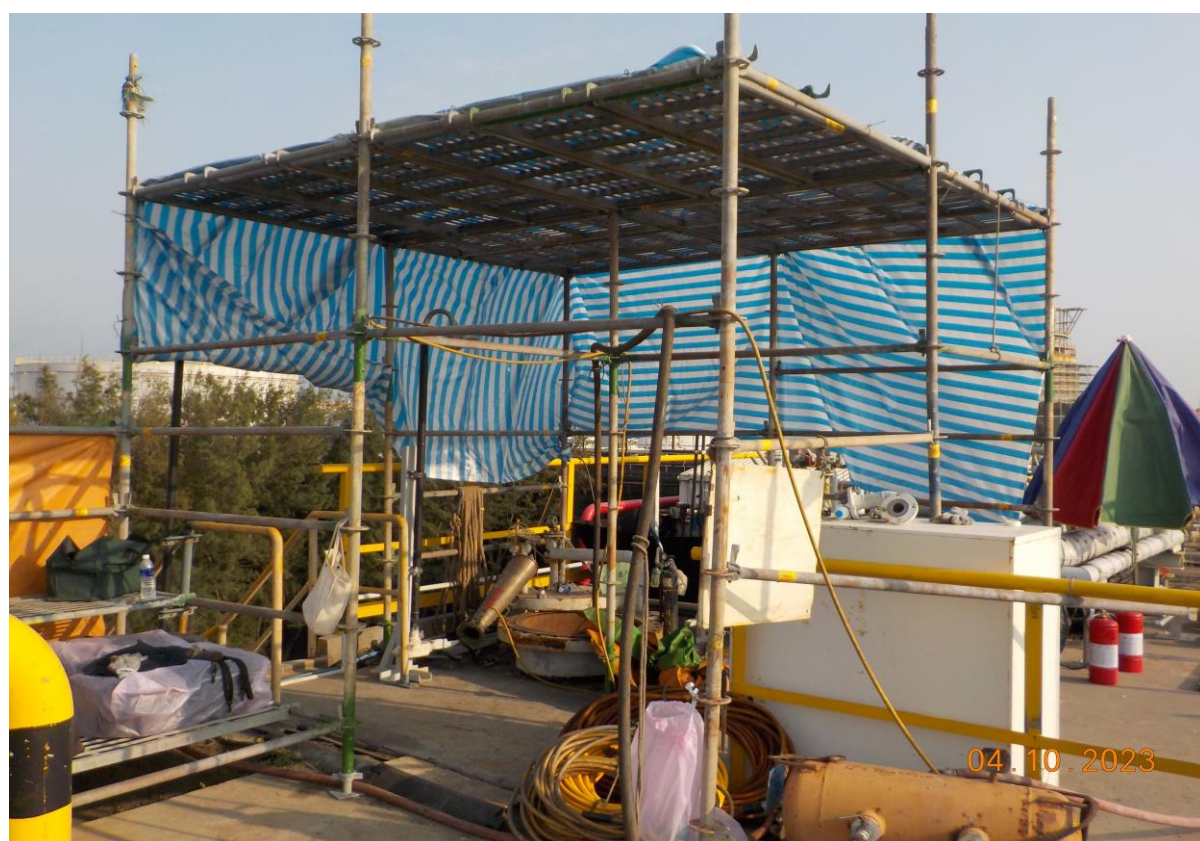
11. 槽外施工架搭設及帆布鋪設情形
