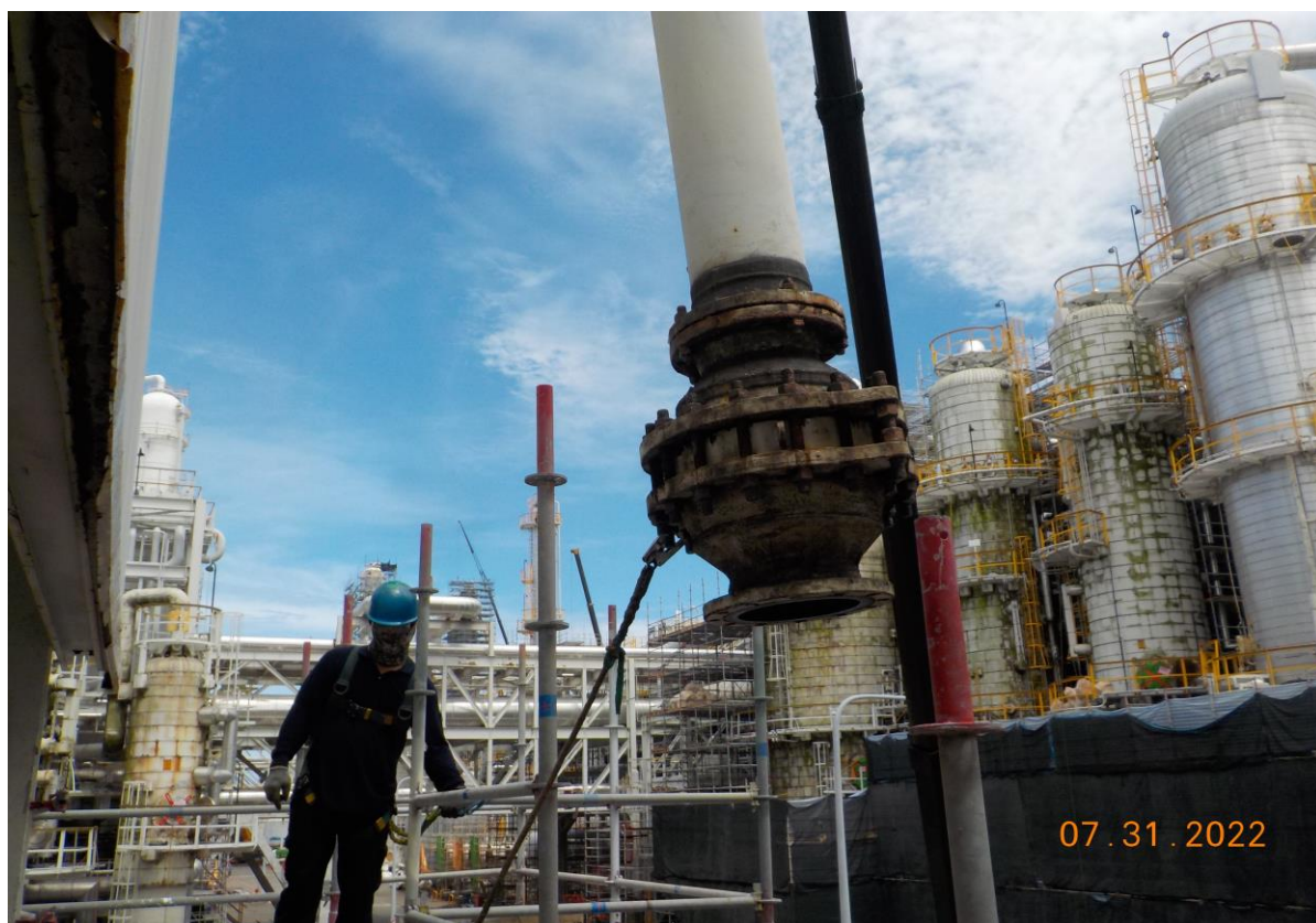
8. 火焰捕捉器移除之情形
