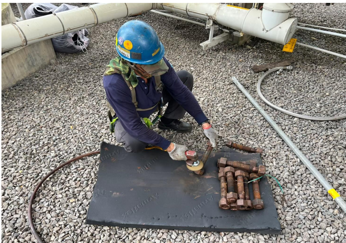
10. 人孔螺絲整理情形
