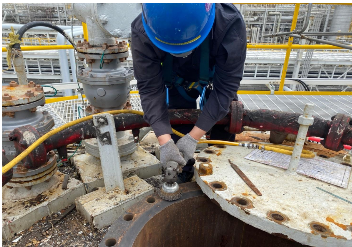
10. 人孔復原前法蘭面整理
