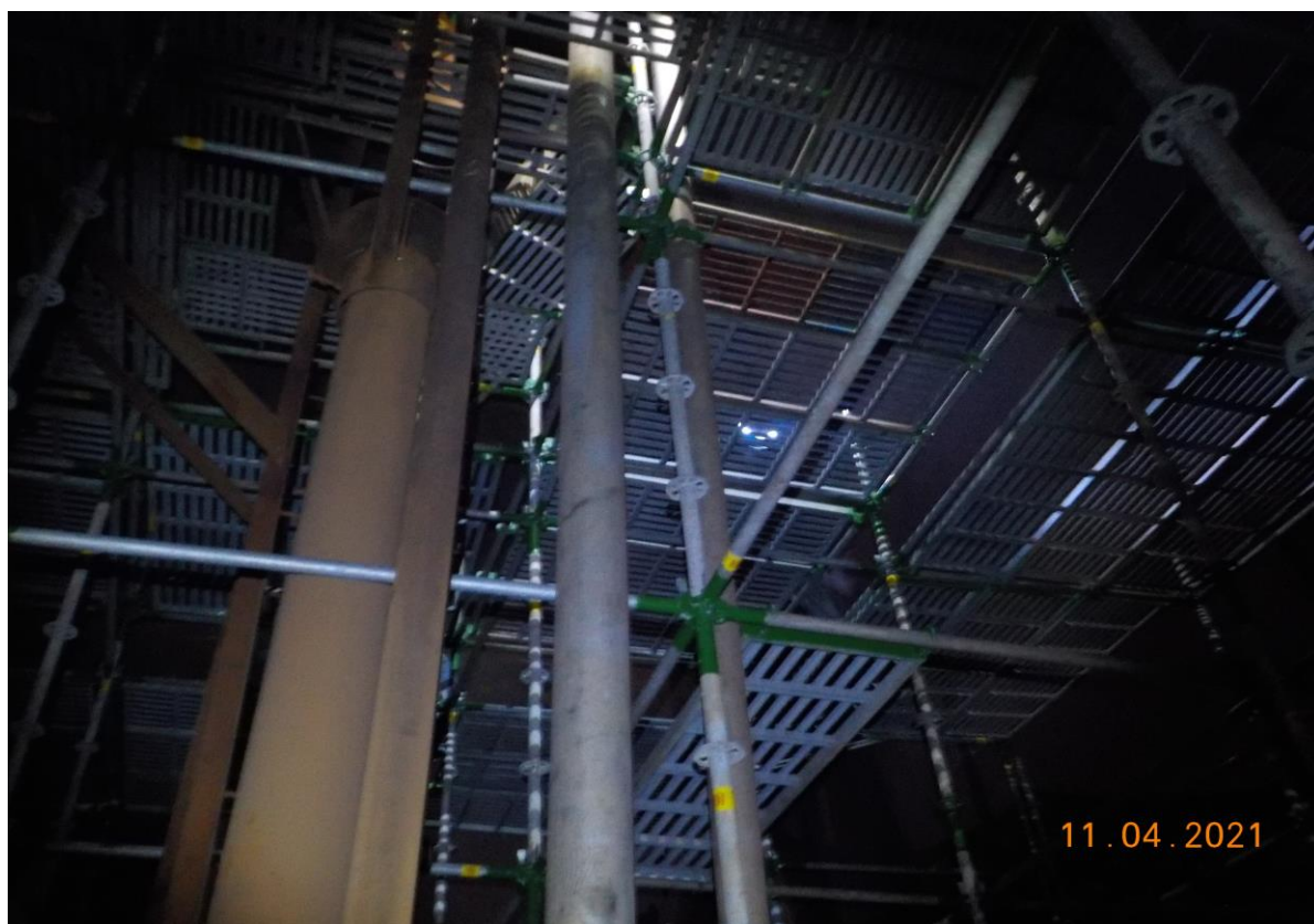
4. 槽內搭架作業情形(2)
