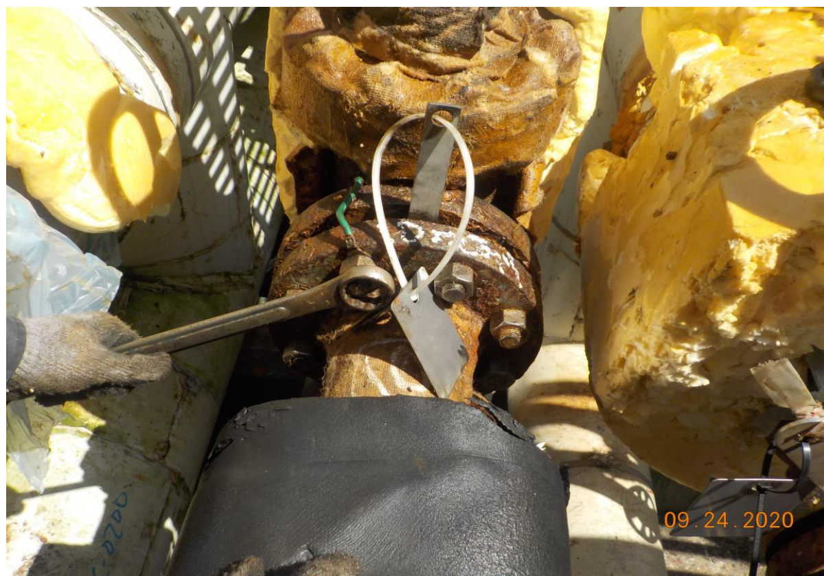
3. 插盲板作業(3)
