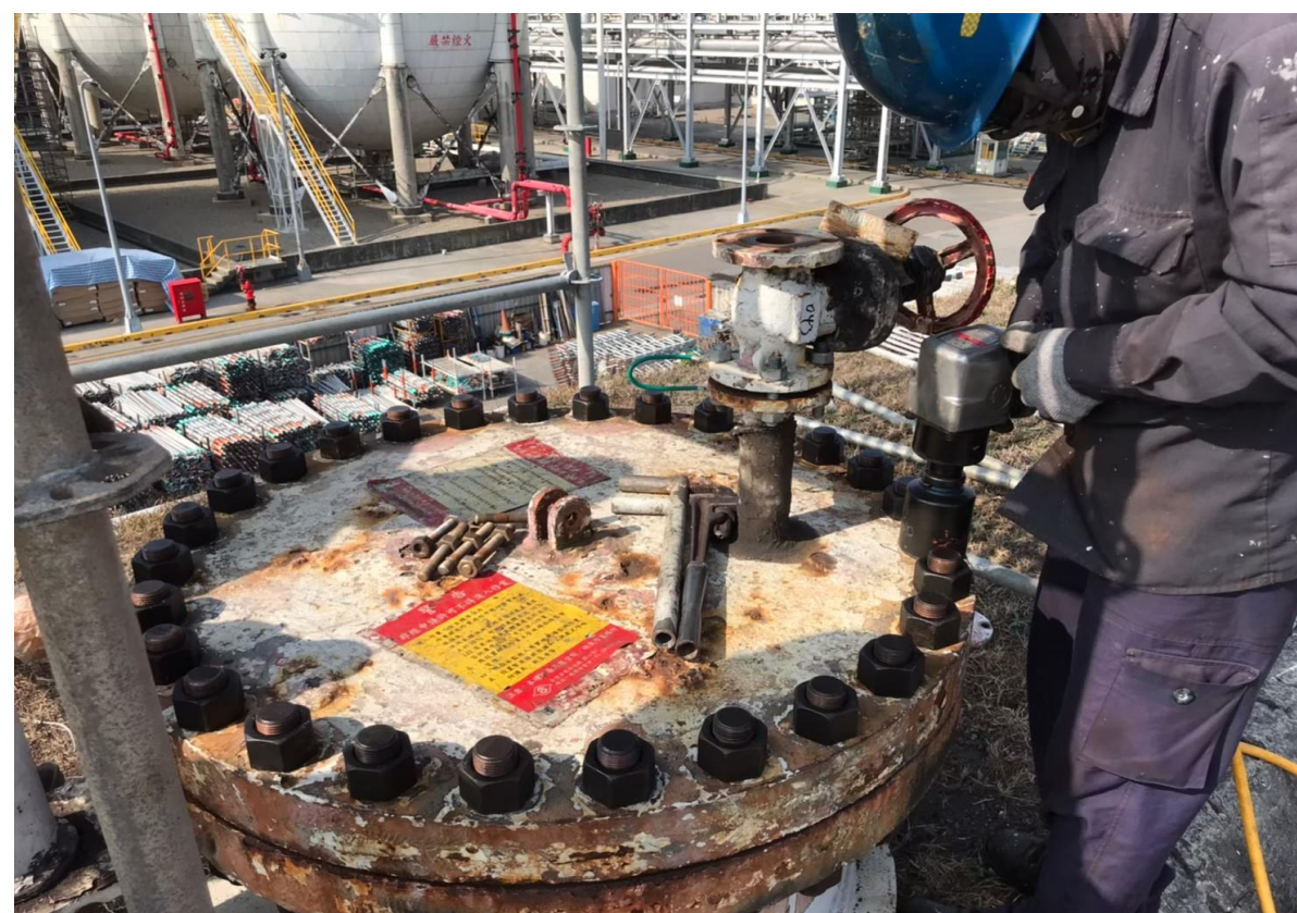
14. 人孔復原之情形(2)
