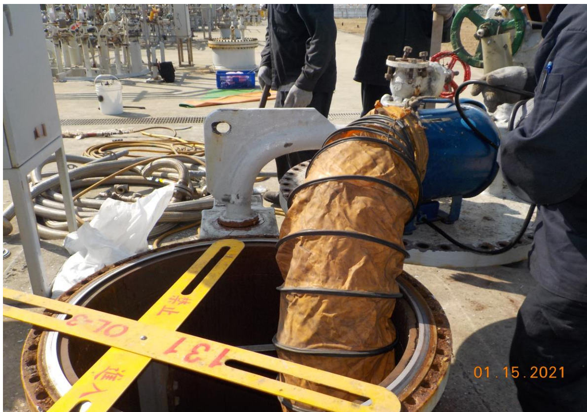
5.通風設備定位情形
