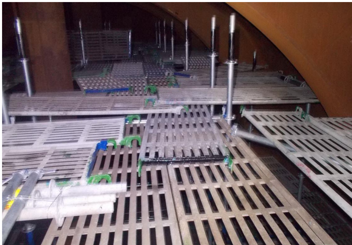
9. 槽內搭架作業情形(3)
