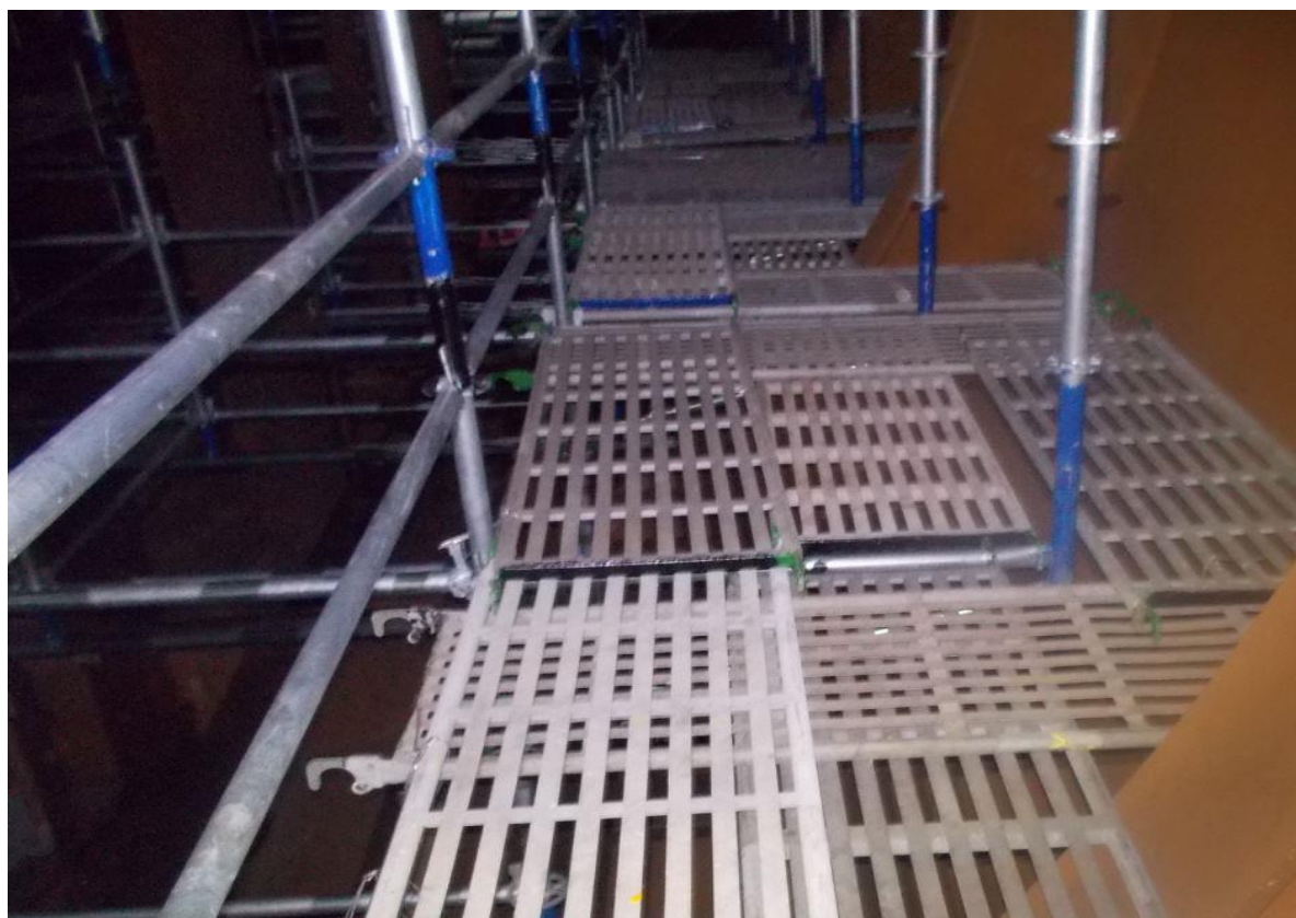
8. 槽內搭架作業情形(2)
