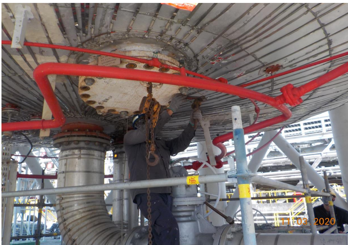
2. 開人孔作業
