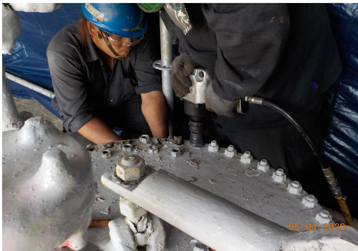
4. 開人孔作業(2)
