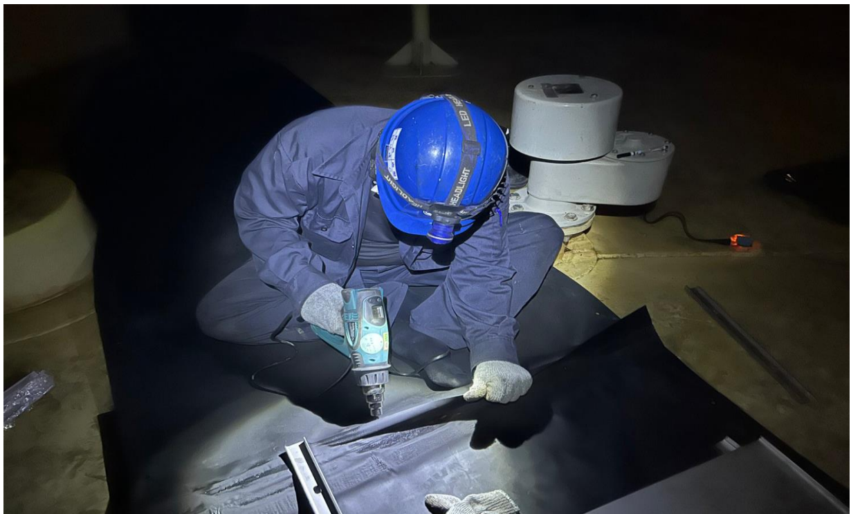
安裝封帶加熱接合情形(10)
