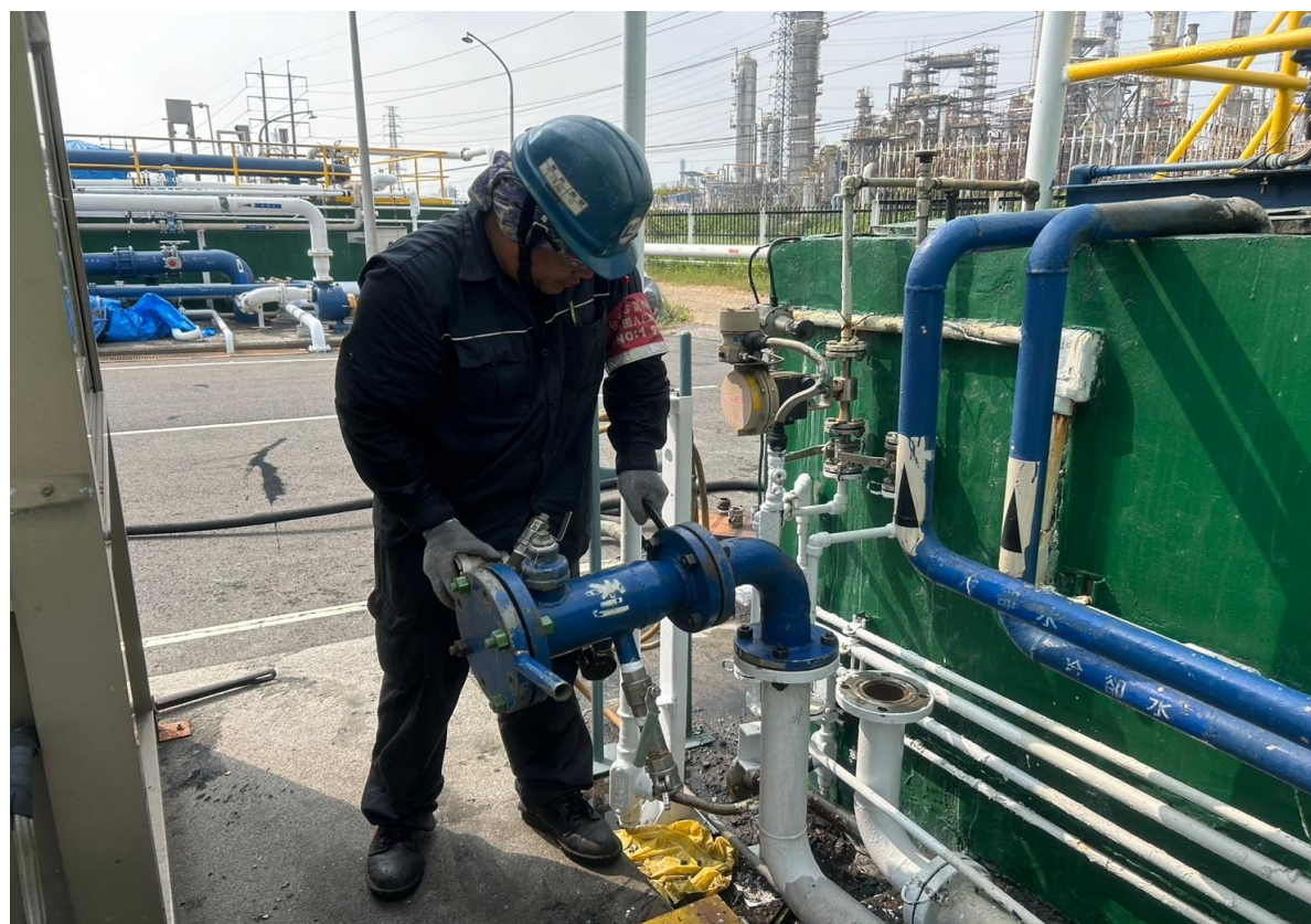
6. 接收段安裝作業
