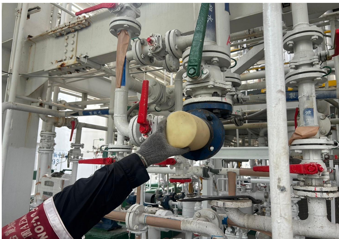
8. B 管海綿 PIG 安裝情形
