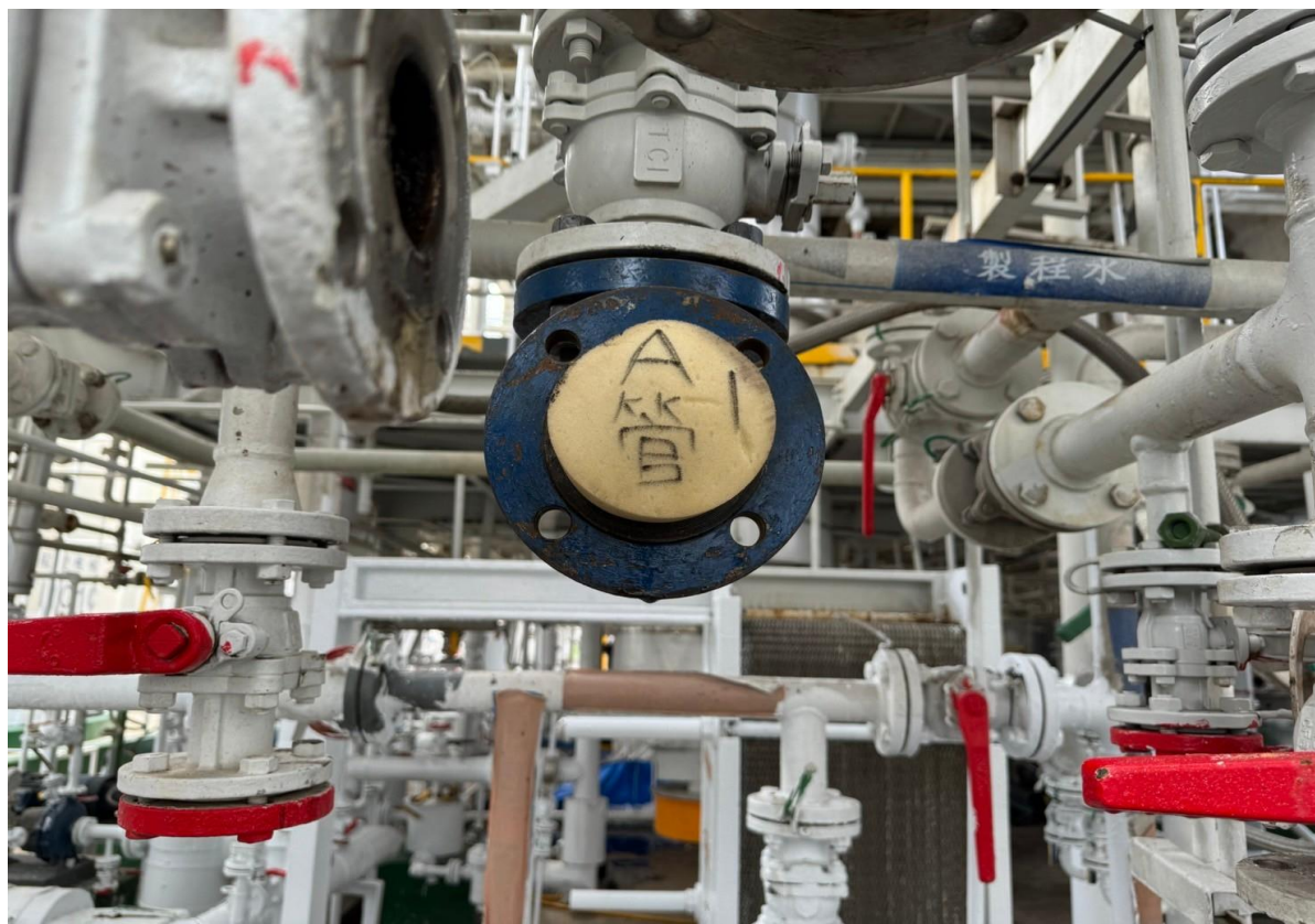
9. A 管發射段安裝 PIG 情形
