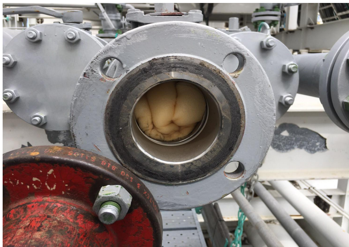
4. 3"PIG 海綿安裝之情形(2)
