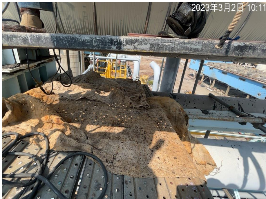
3. 防火毯鋪設情形
