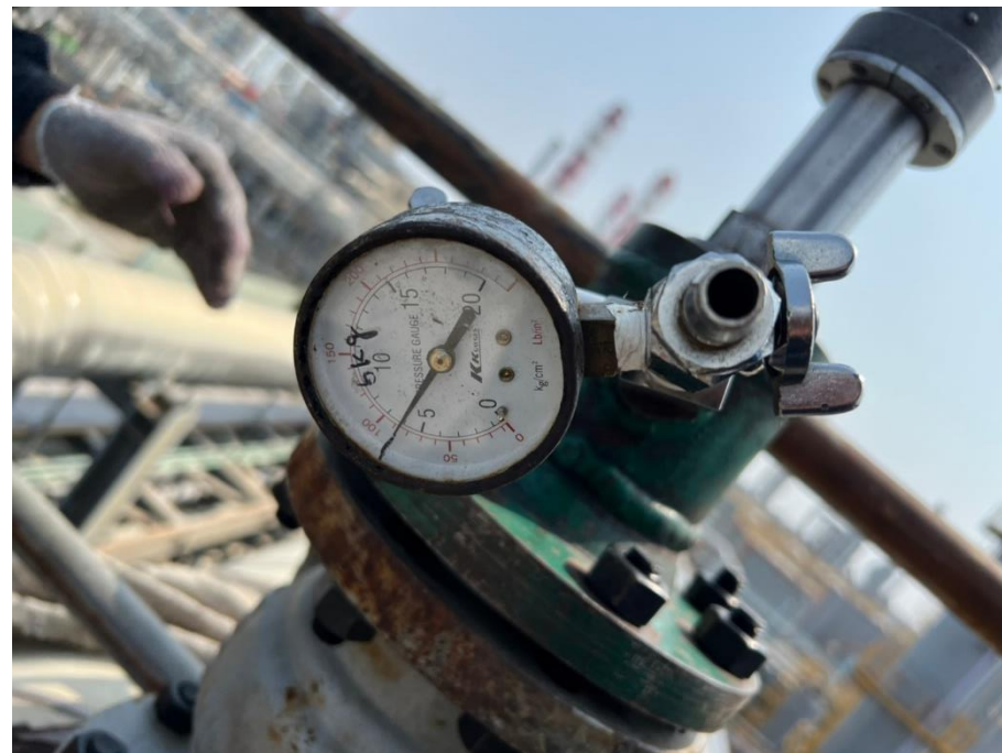
8. 試壓抓漏
