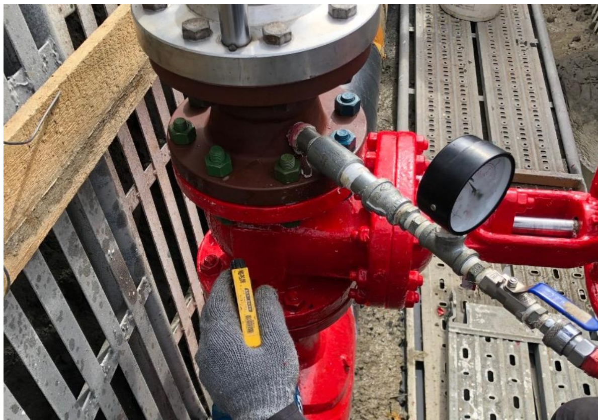
1. 6"試壓抓漏
