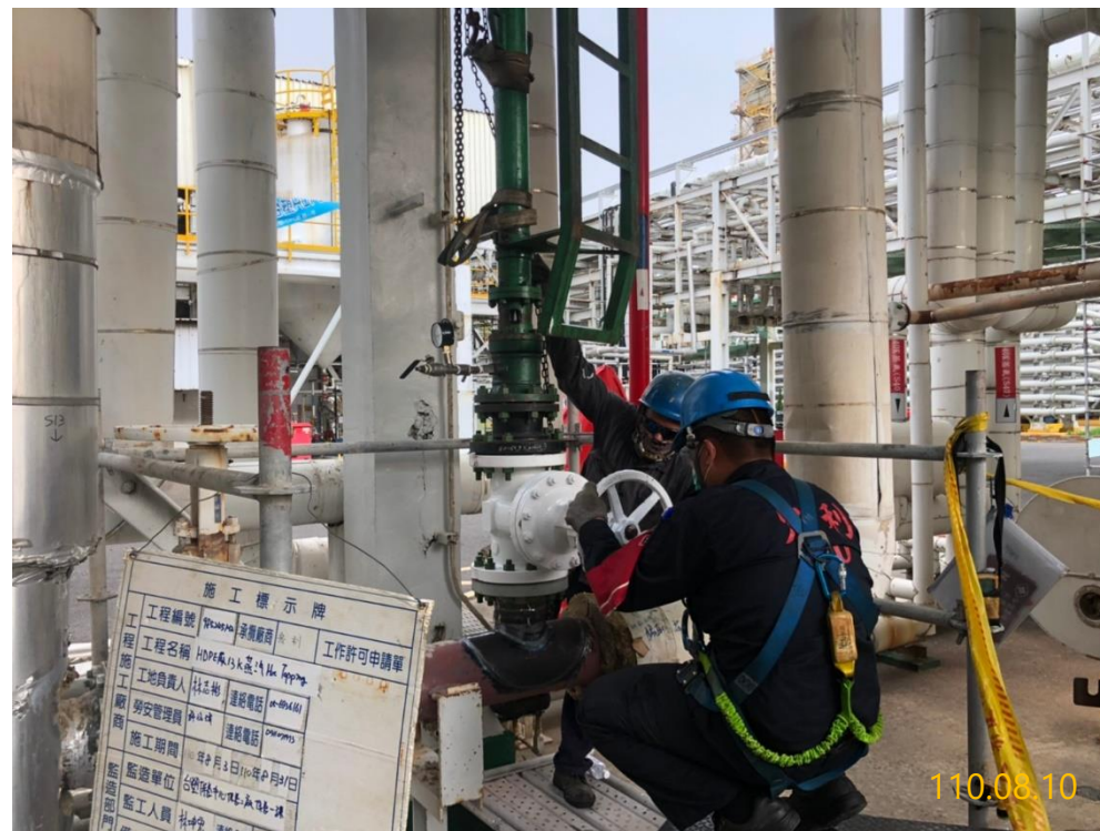
10. 開孔完成閘閥關閉
