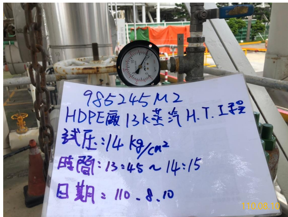
8. 試壓後(14kg/cm 2 持壓半小時)
