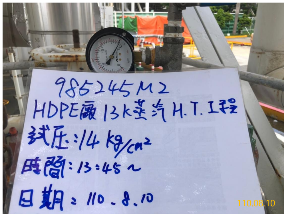
7. 試壓前(持壓 14kg/cm 2 )
