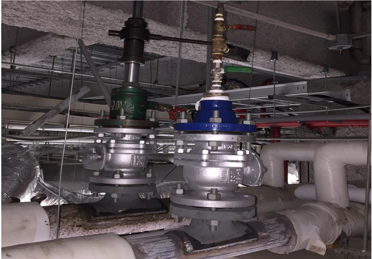
3. 安裝機具及盲法蘭進行試壓作業
