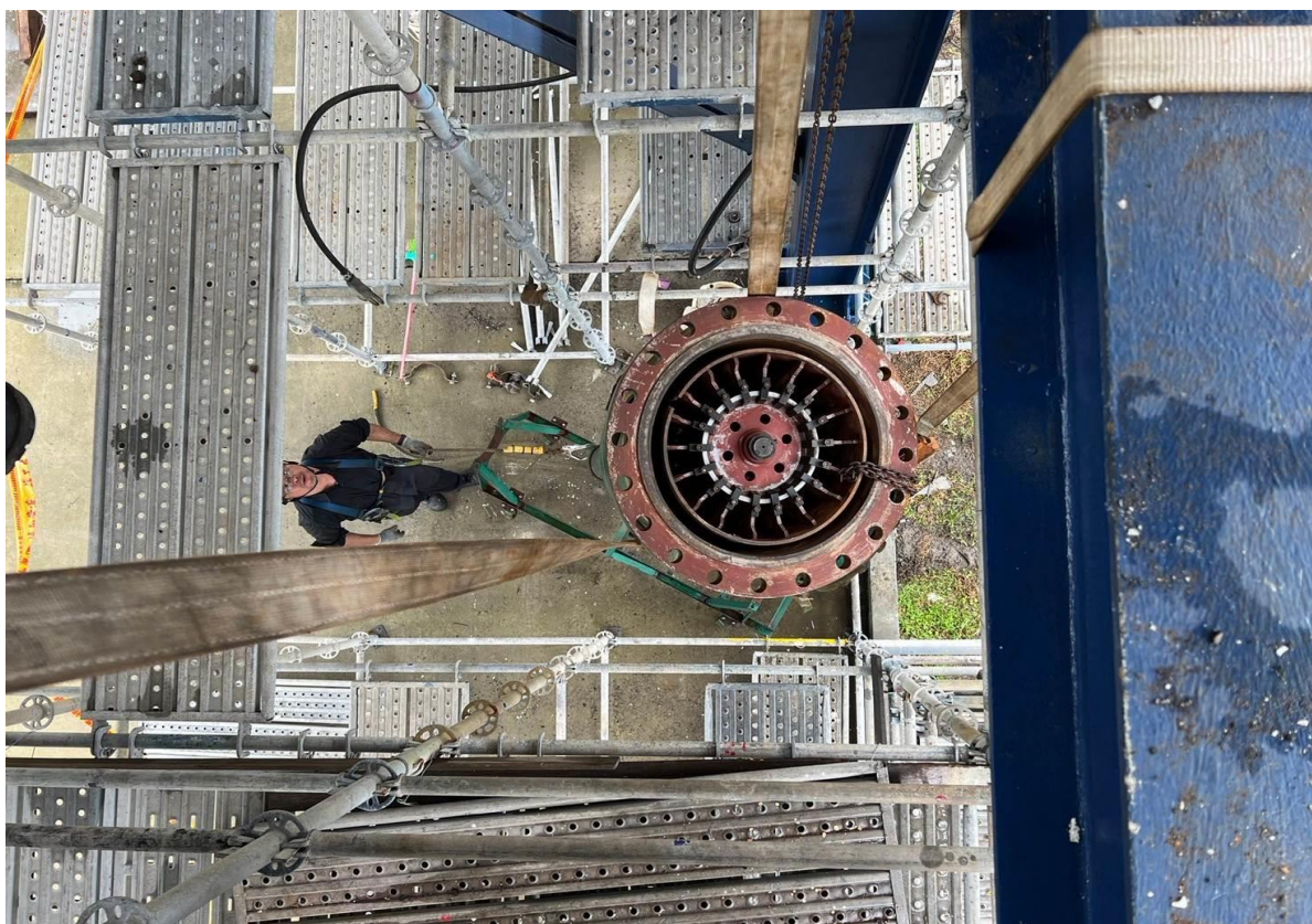
6. 阻斷機具吊裝作業
