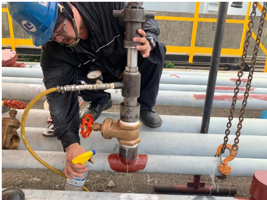
5. 閥件及開孔機具安裝作業
