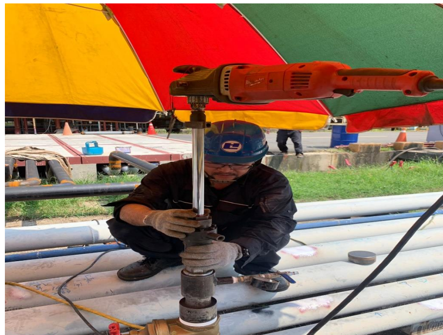
8. 人員執行開孔作業
