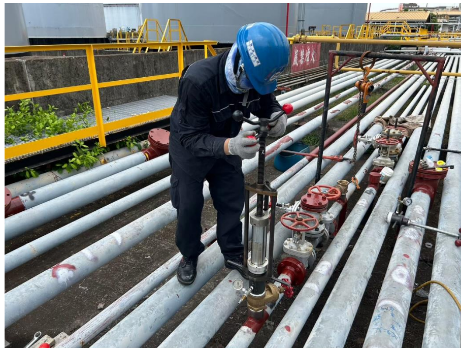
14. 管線增設閥件及三通
