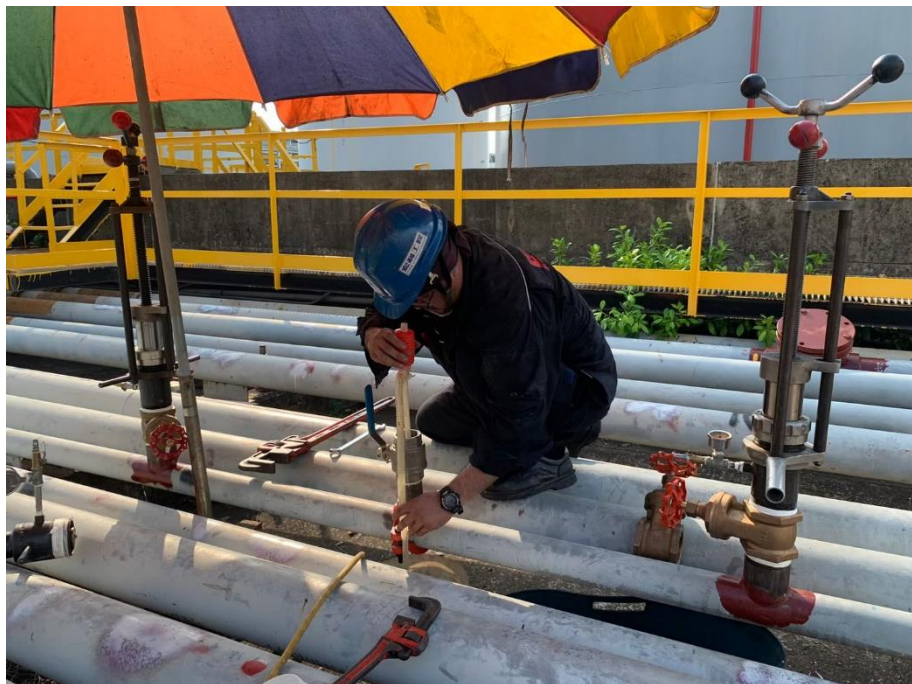
11. 管線內部油品抽油作業
