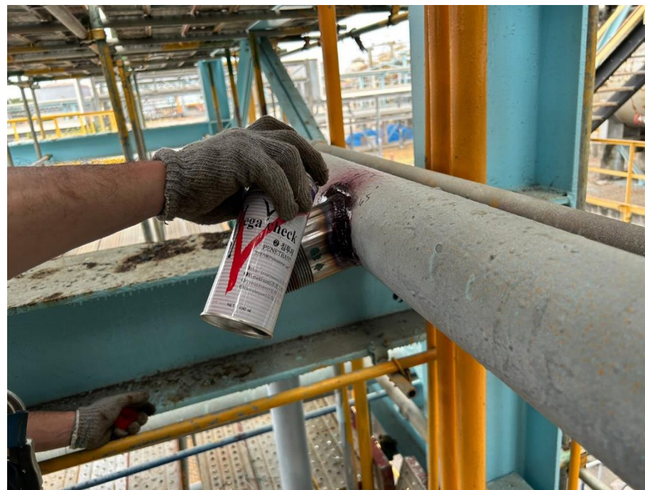
6. PT 液滲檢測左側
