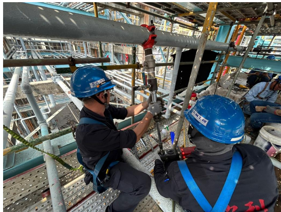
12. 人員安裝夾式開孔進行開孔作業(2'')
