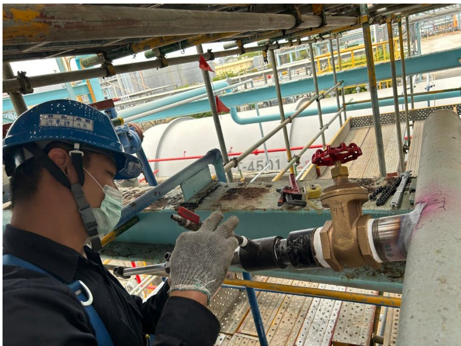
17. 人員進行阻斷作業
