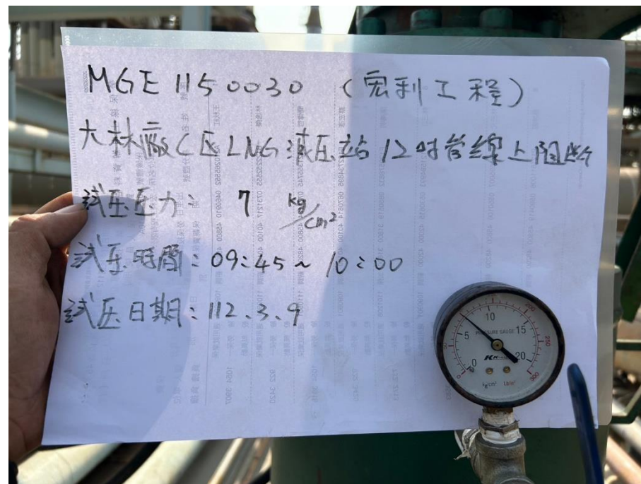
8. 試壓作業
