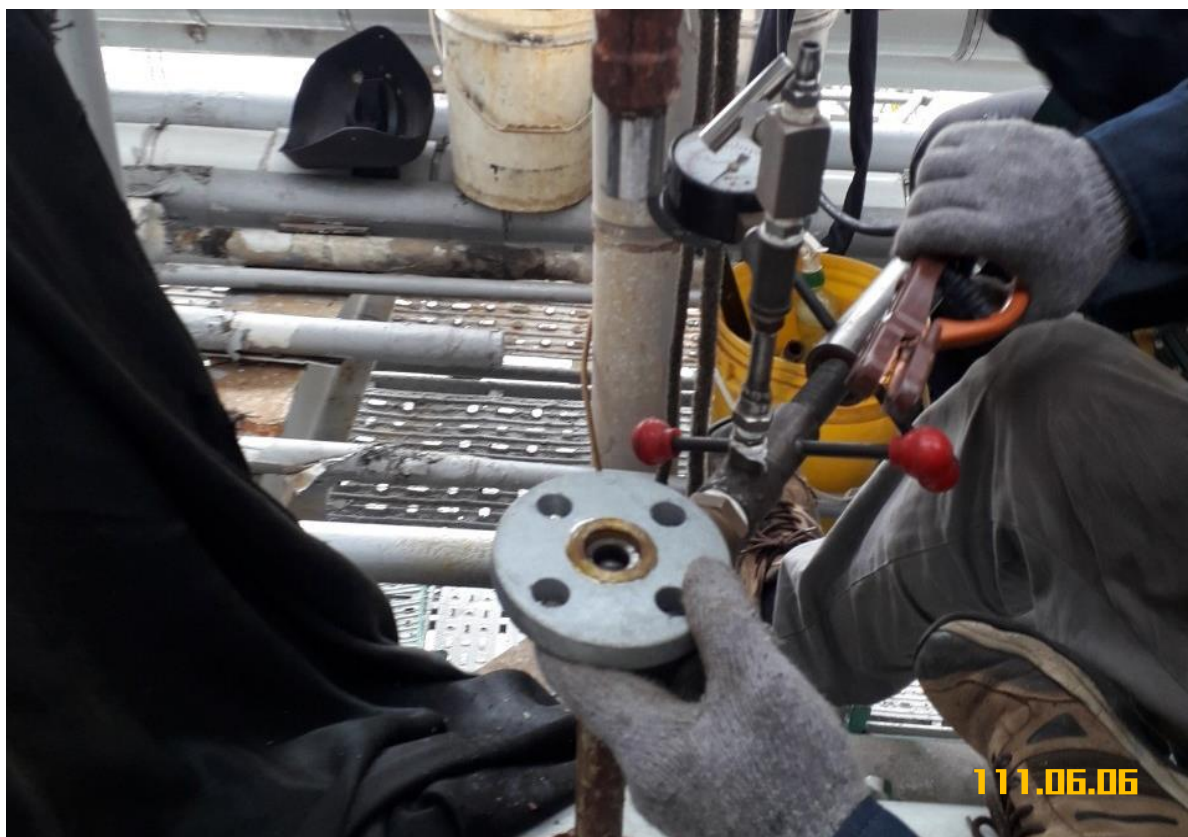
6. 阻斷後進行切管焊接法蘭
