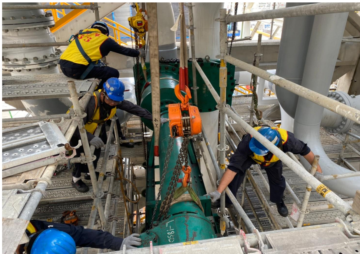
1. 開孔機及夾板閥安裝後進行斷管作業
