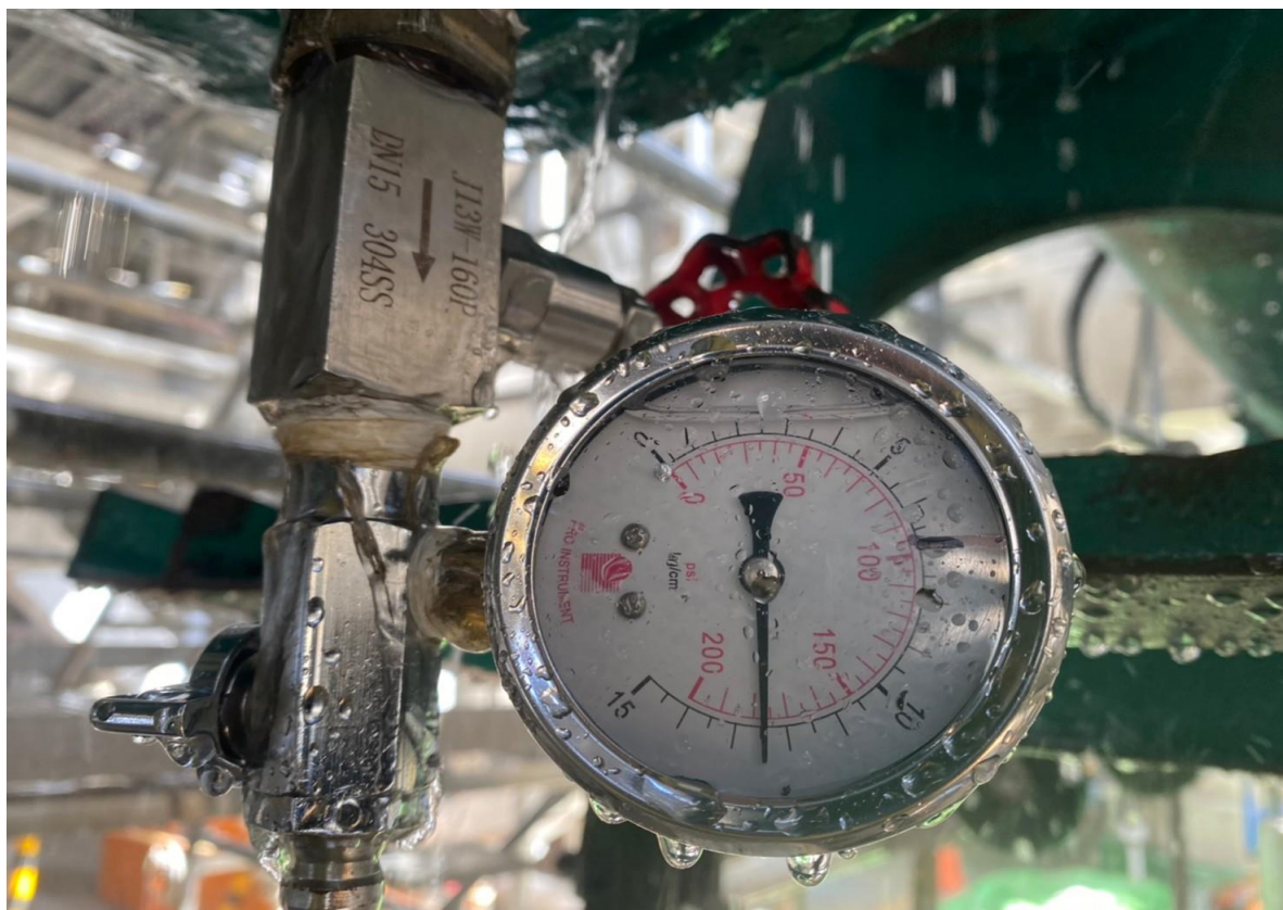
3. 第二口 夾板閥及開孔機安裝後試壓作業
