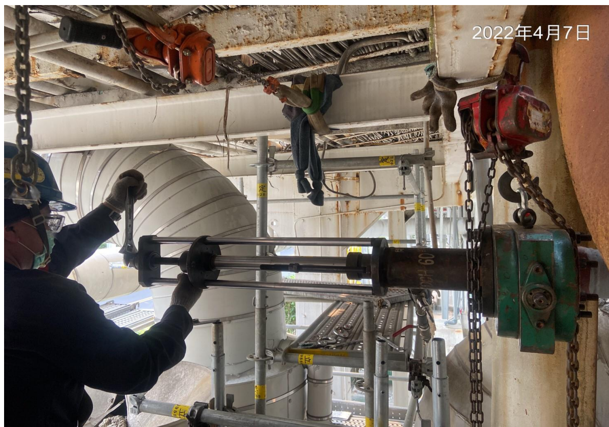
28. 安裝阻斷器進行阻斷作業
