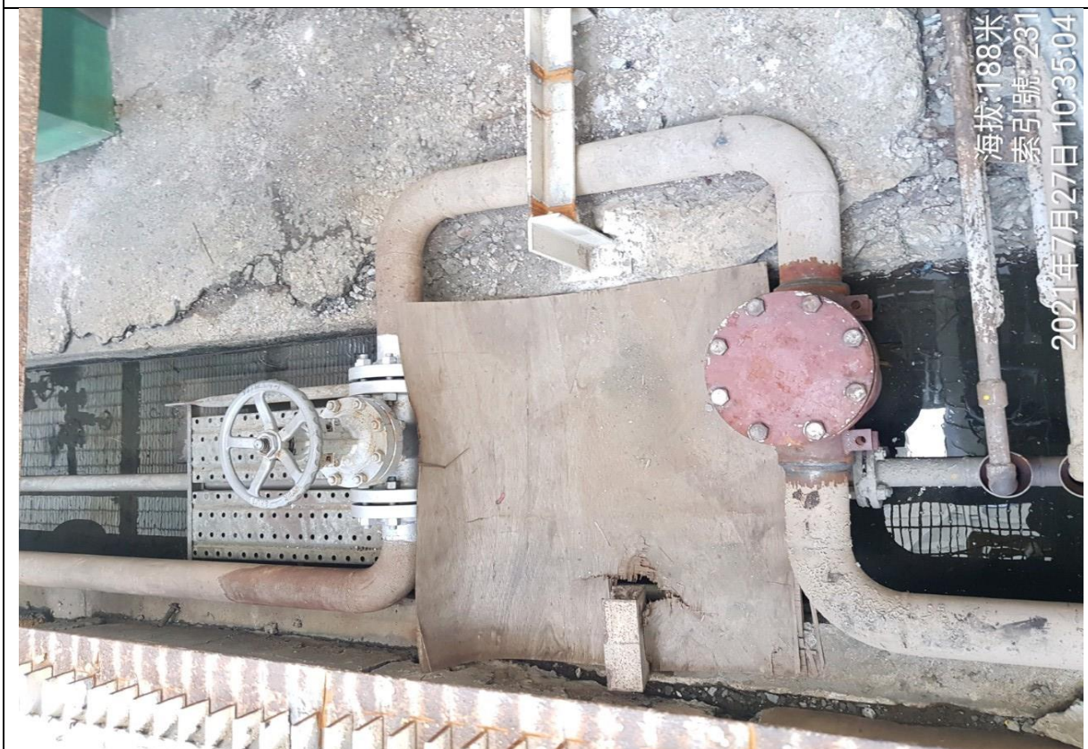
6. 4"阻斷增設閥件完成
