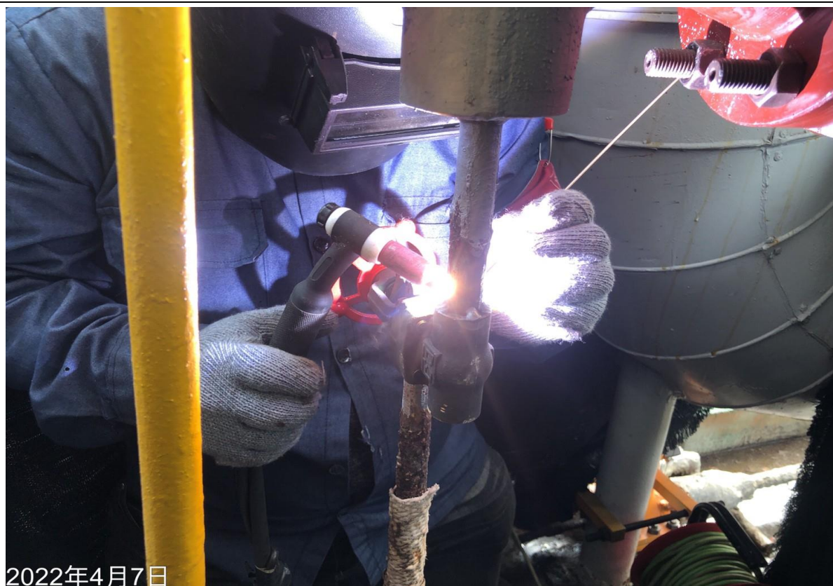
23. 阻斷後新增閥件
