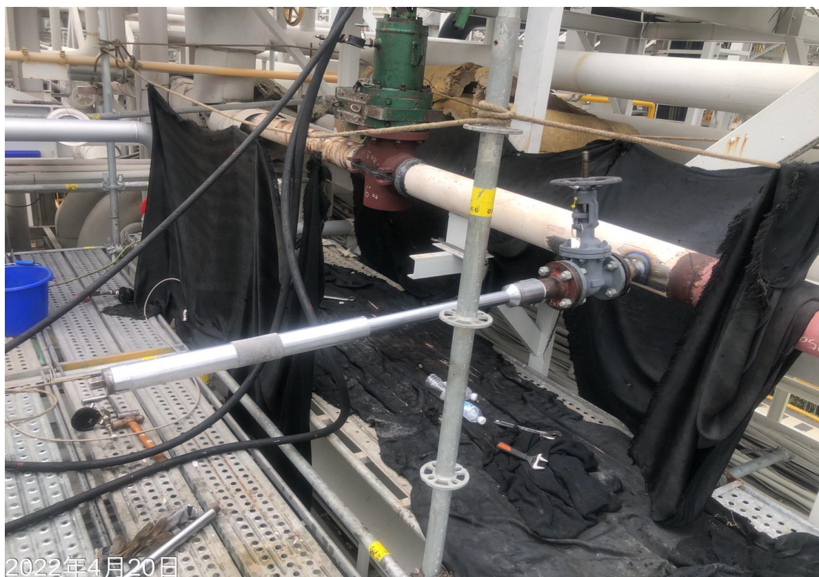
25. 下游處進行開孔作業，以利排壓確認
