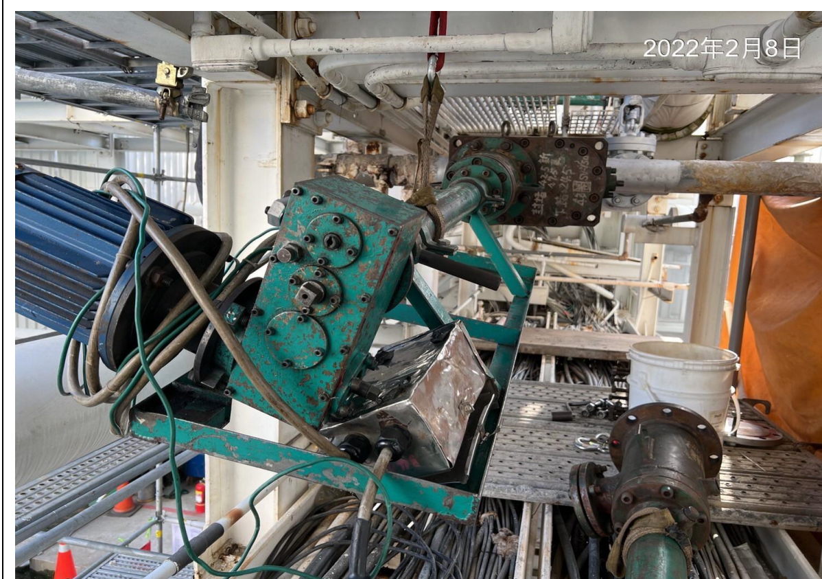
12. 安裝夾板閥及開孔機進行斷管作業(4'')
