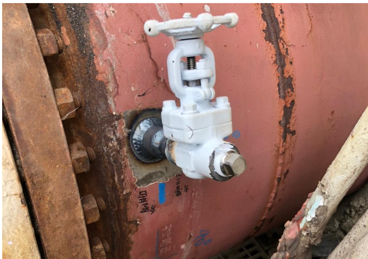
28. 開孔完成
