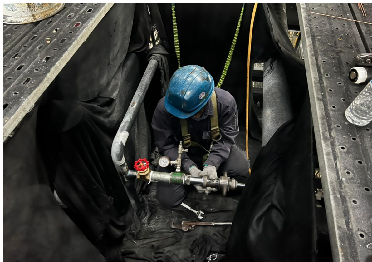
20. 人員安裝開孔機進行開孔作業(2’)
