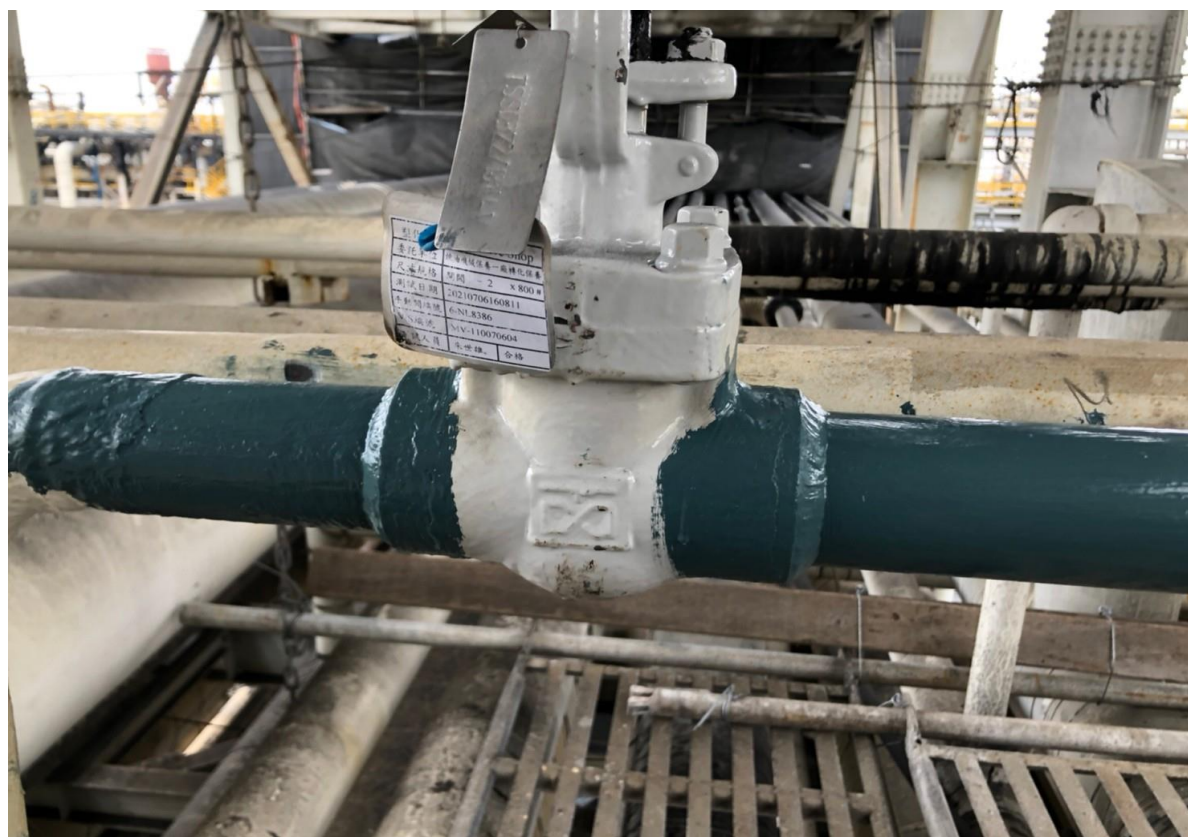
16. 阻斷新增隔離閥情形(1")
