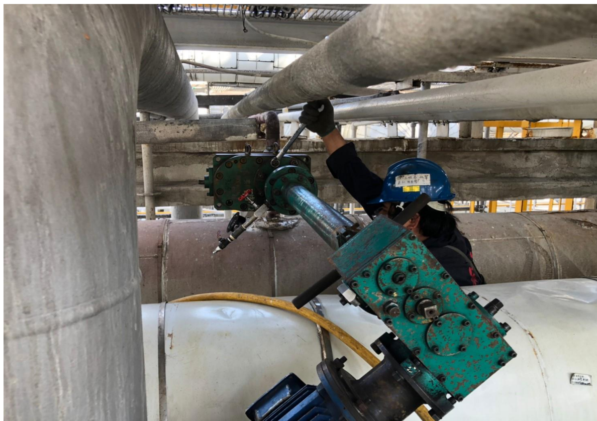
31. 人員安裝開孔機後進行斷管作業
