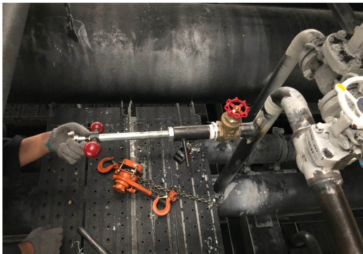
23. 下堵作業
