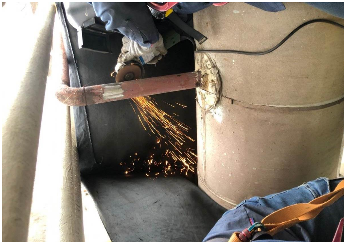
29. 管線研磨
