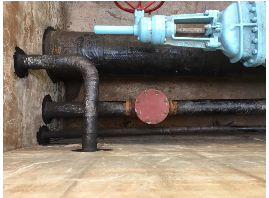
16. 施工完成，安裝盲蓋(2)
