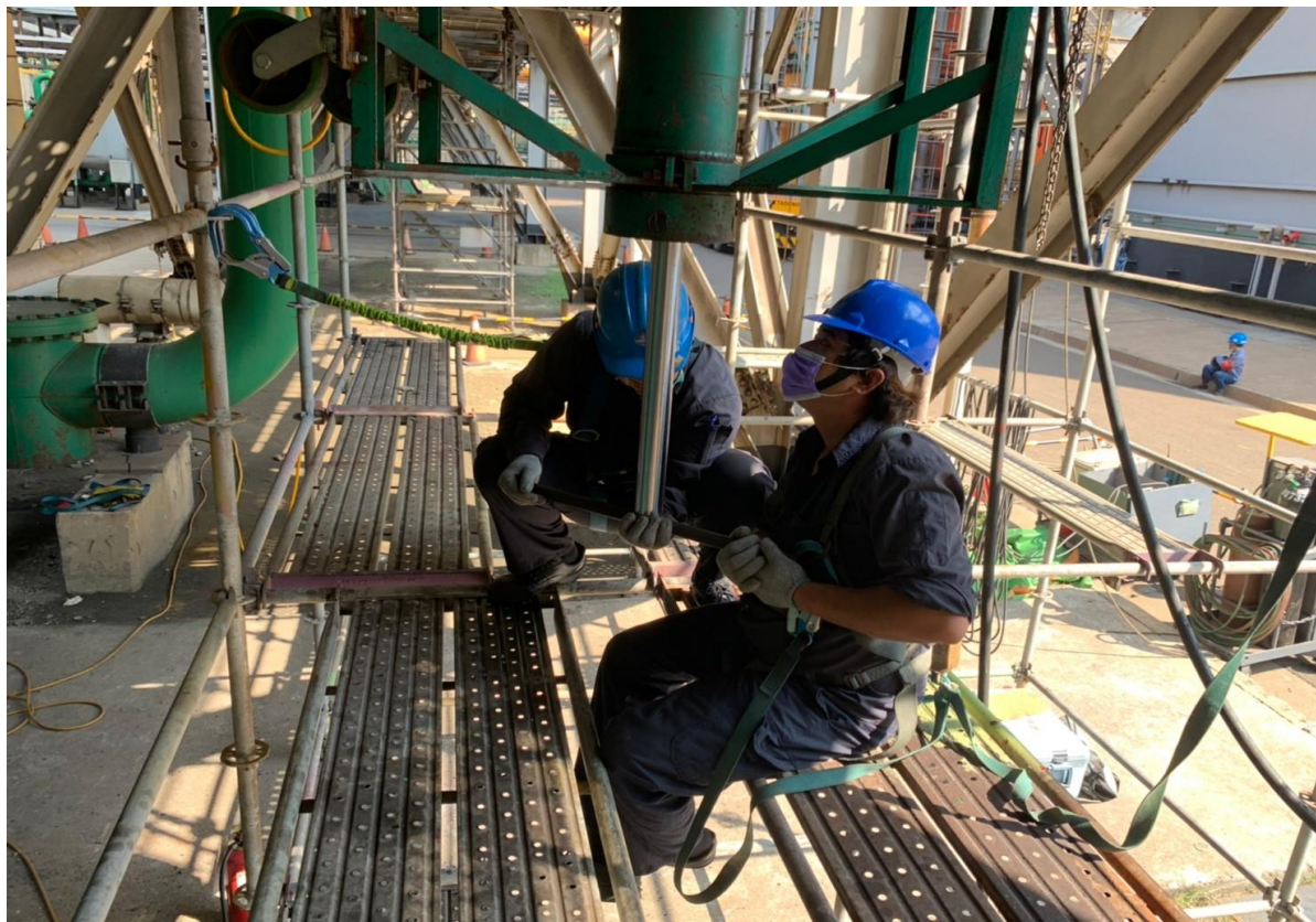
5. 安裝阻斷器後進行阻斷作業
