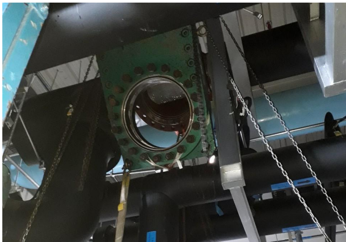
3. 夾板閥吊裝作業
