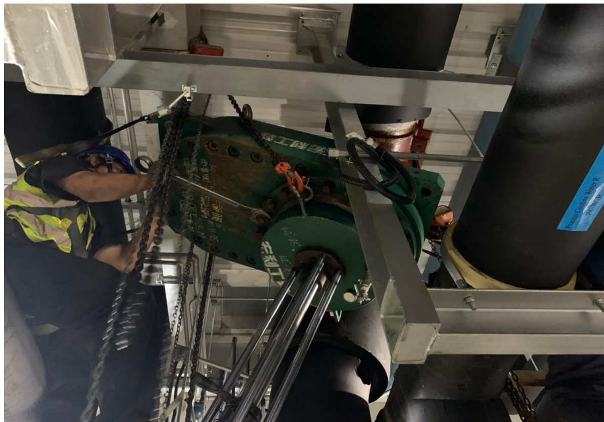
20. 下堵安裝作業
