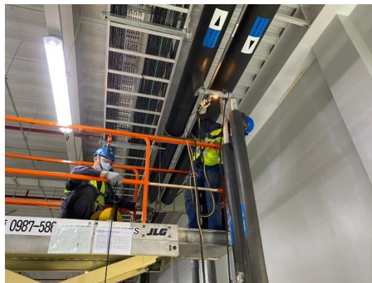
阻斷鞍座焊接作業
