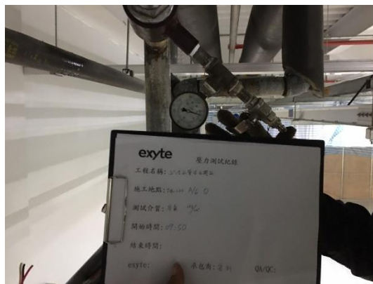
開孔前進行試壓作業
