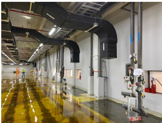
管線施工前
