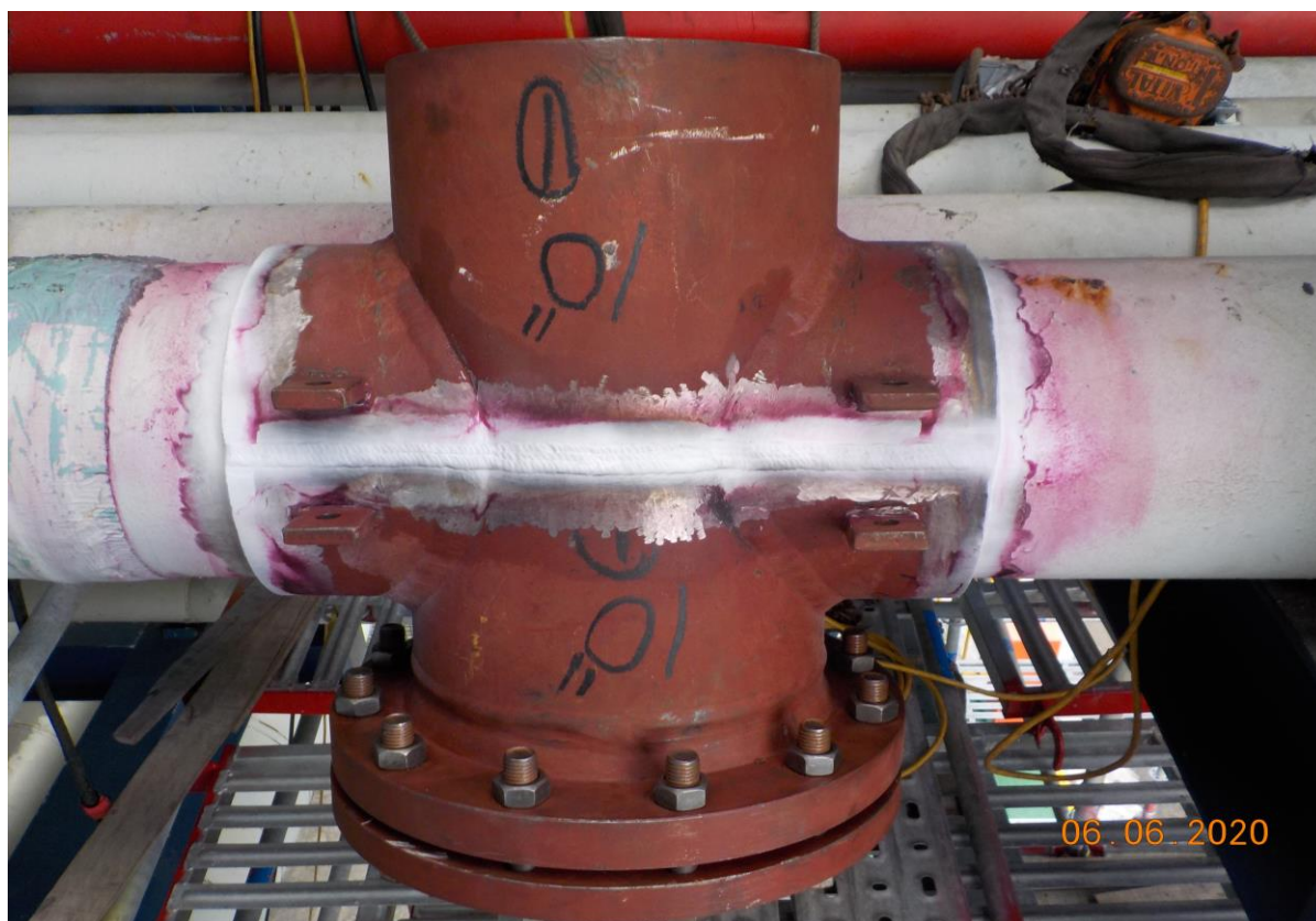
12. 管線線上開孔及阻斷完成
