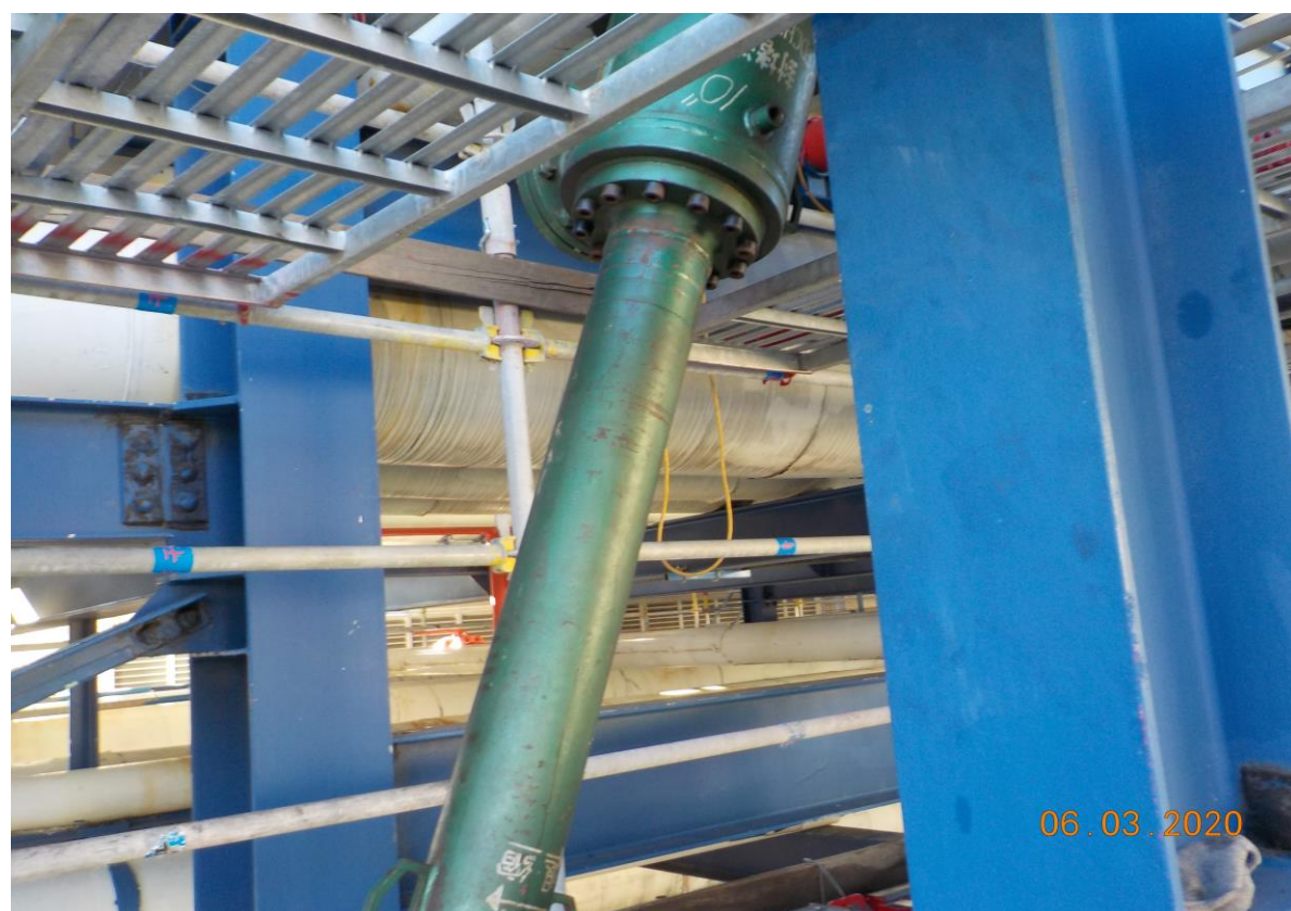
6. 斷管完成進行阻斷機具安裝
