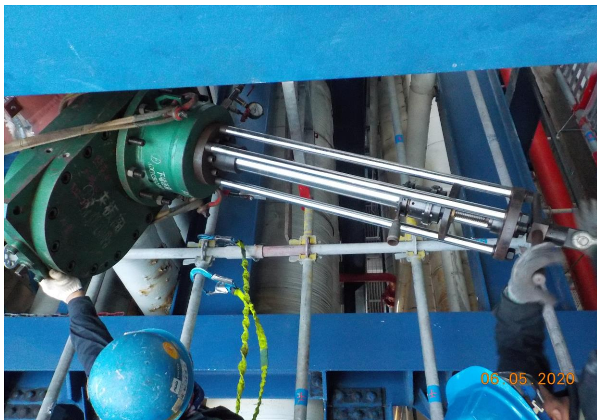
11. 閥件新增完成，進行下堵作業
