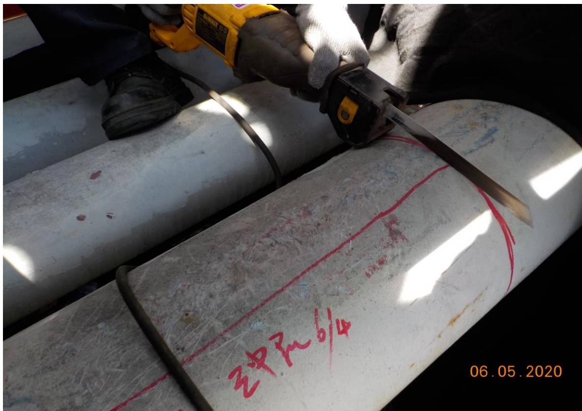
7.阻斷完成後進行無火花切割作業
