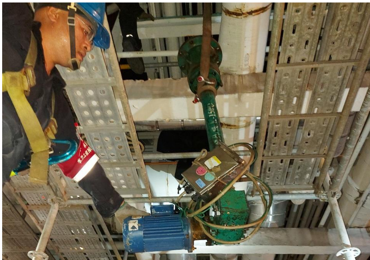
3. 開孔機安裝後進行斷管作業
