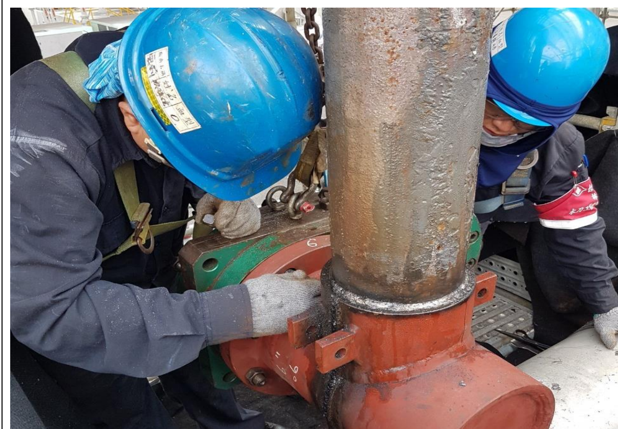
12. 6"阻斷模具焊接後安裝夾板閥作業
