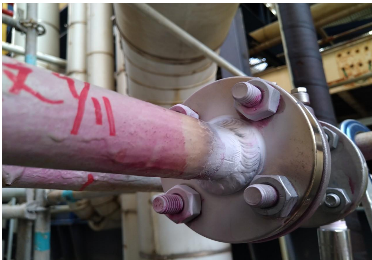
8. 法蘭焊接處液滲(PT)檢查
