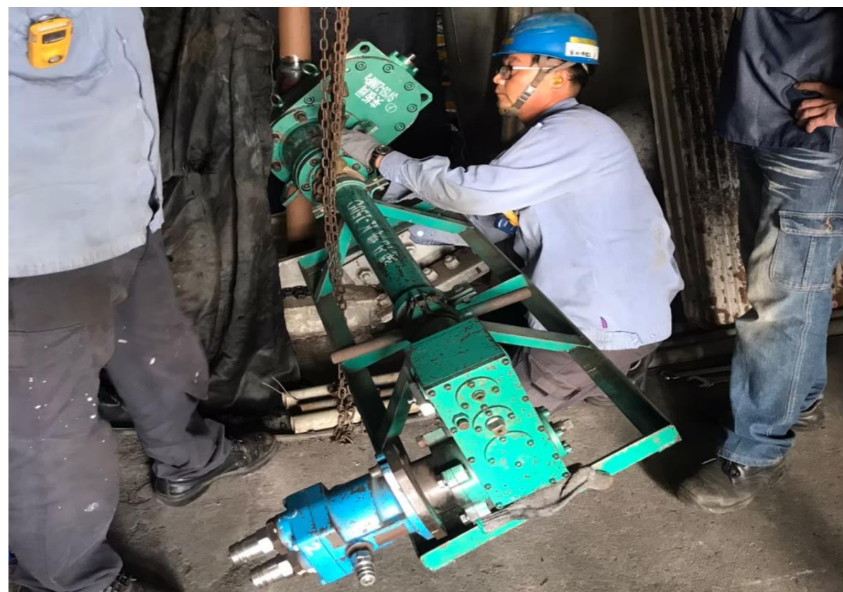
2. 開孔機安裝後進行開孔作業
